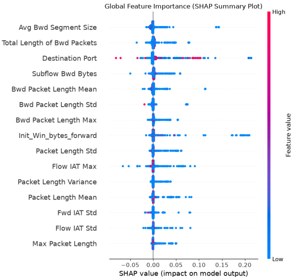
Σχήμα 5.3: Συνοπτικό γράφημα SHAP. Η θέση στον οριζόντιο άξονα δείχνει την επιρροή στο αποτέλεσμα (δεξιά αυξάνει την πιθανότητα "Επίθεσης"), ενώ το χρώμα (μπλε έως φούξια) υποδηλώνει την αρχική τιμή του χαρακτηριστικού.
